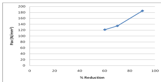
Fig 3.6 Percentage Reduction vs P av graph (m=0.38)
