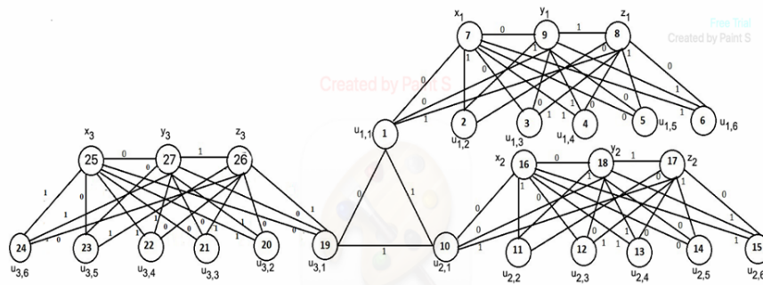
Figure 5'. C (3. (+ Γ(Z 6 )))
