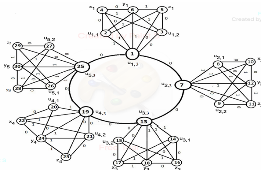
Figure 2. C(5, \Gamma(Z_6) + \Gamma(Z_6))
